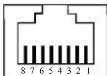
图 10 RJ45 接口
