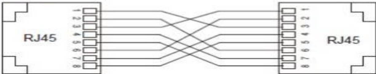
图 7 10/100/1000Base-T(X) RJ45 接头直连线、交叉线互连
